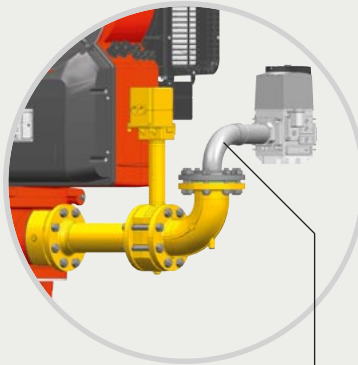
Gasarmatur für Zweigas- brenner entsprechend Armaturen- auswahl Beispiel: Geflanscht
