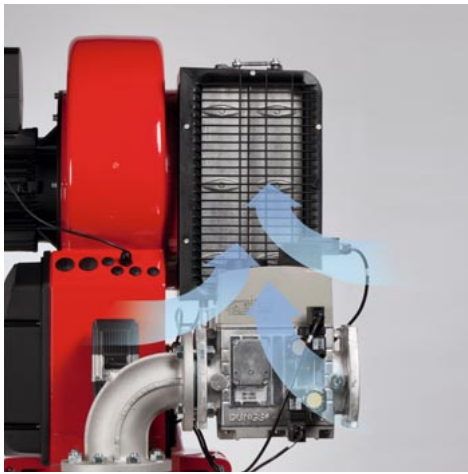
Das Gasabsperrrventil ist optimal positioniert und durch die Nähe zum Ansauggehäuse zusätzlich gekühlt
