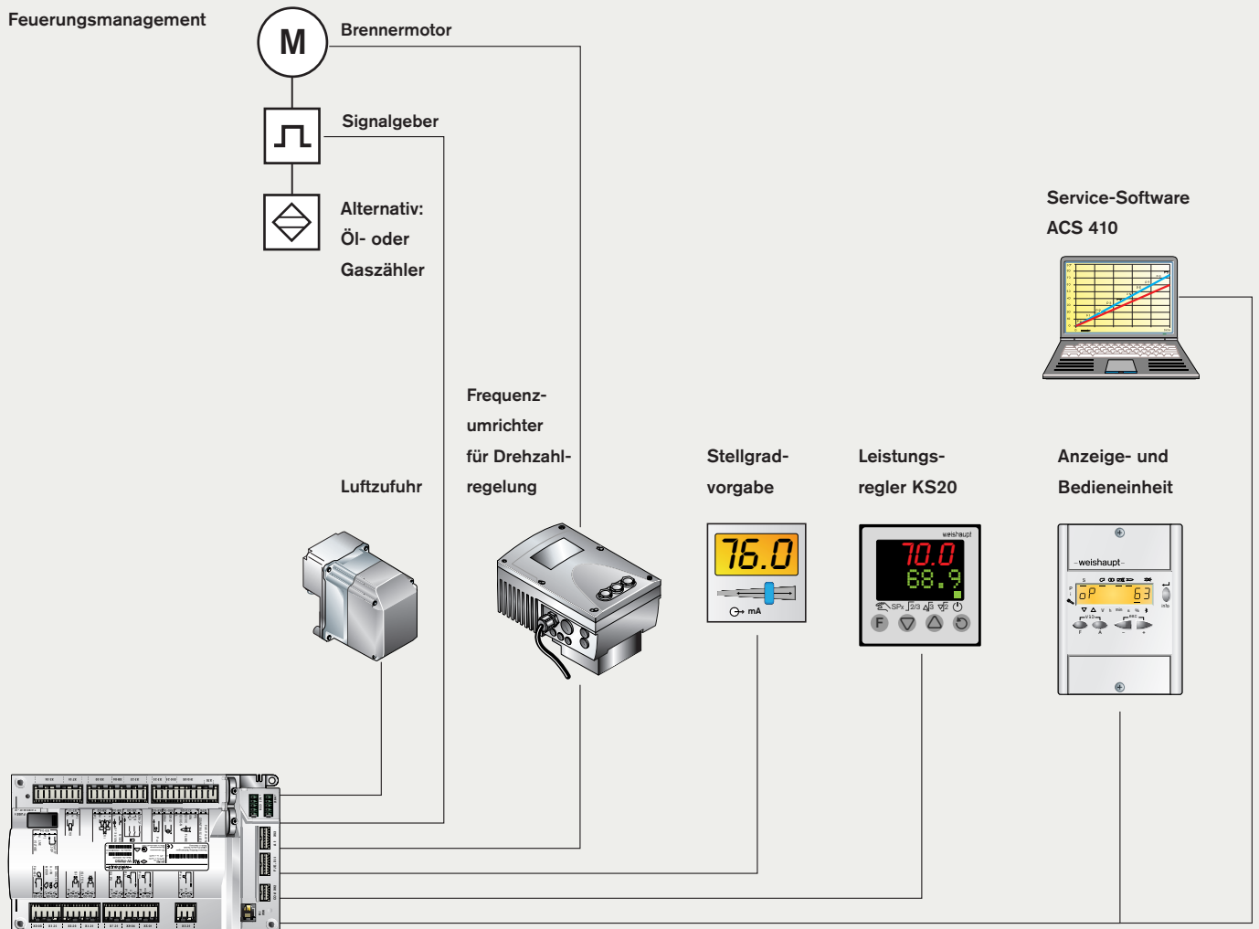
Feuerungsmanager W-FM54 und Umschaltbox
