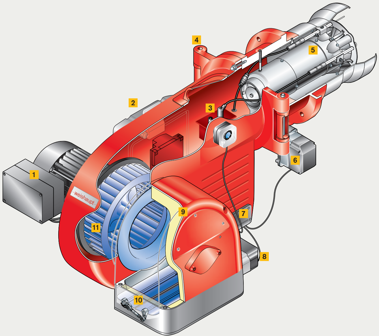
WM-G30 Ausführung ZM-3LN
