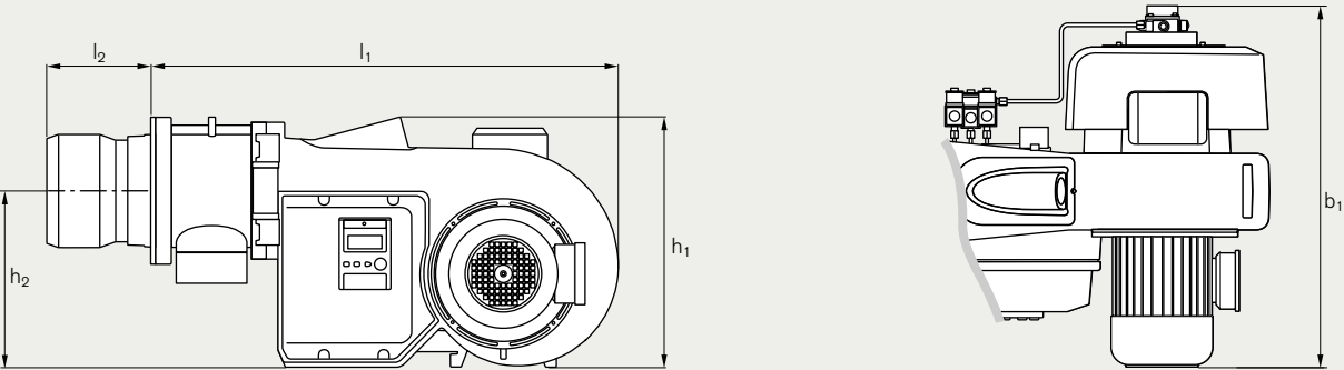
Abmessungen - Ausführung Standard / LN
