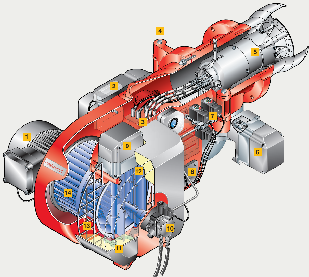
WM-GL10 Ausführung ZM-T
