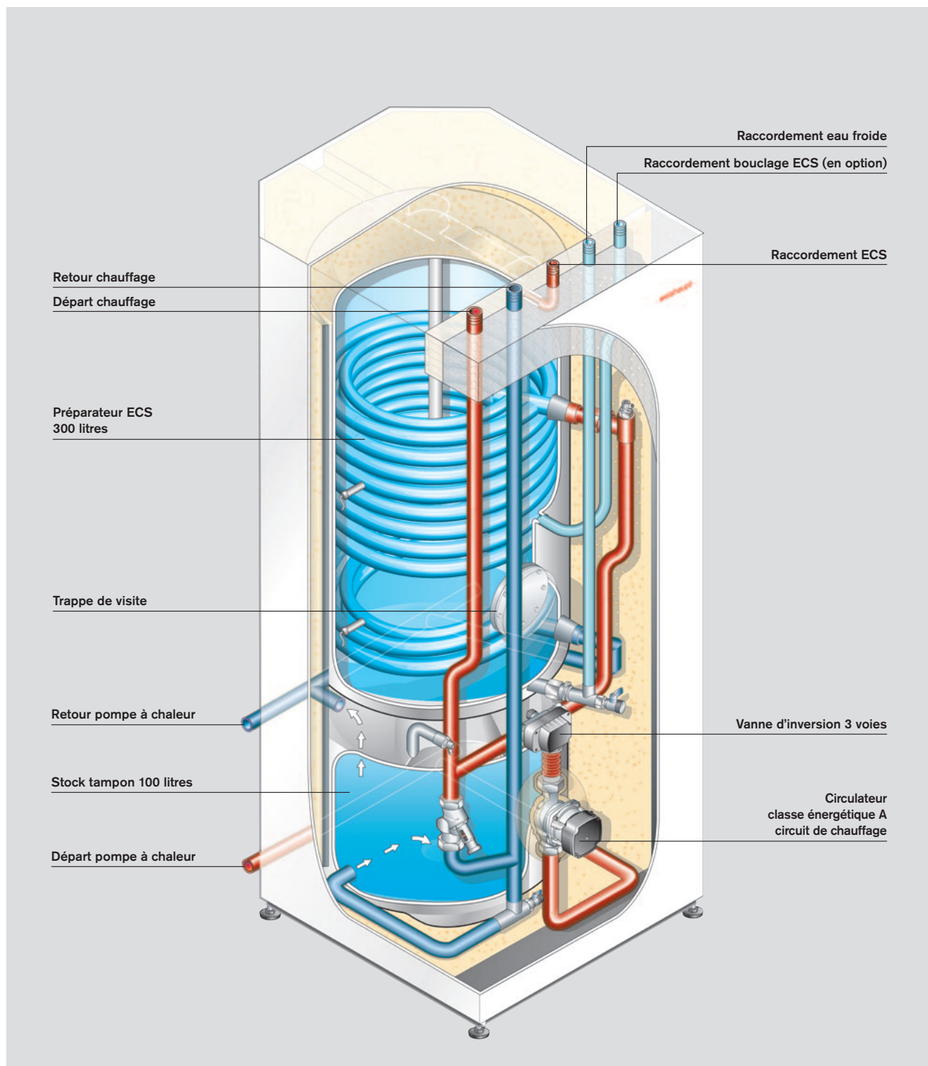
Préparateur multifonction Weishaupt WKS 300 / 100 LE / Unit / Bloc / C pour pompes à chaleur bi-bloc
