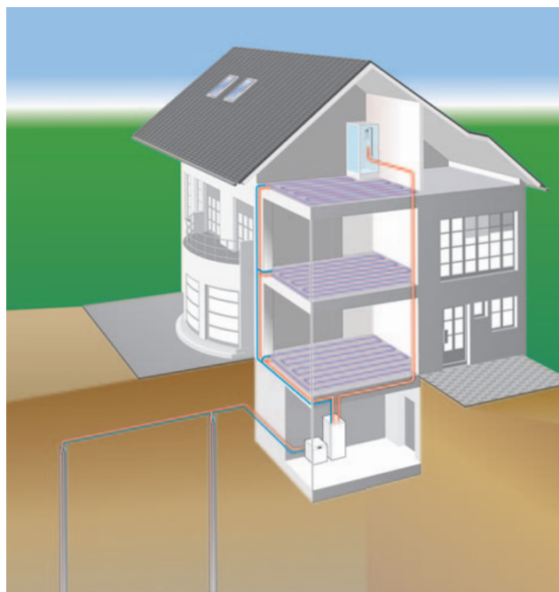
Sondes géothermiques verticales
