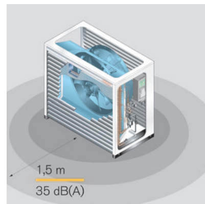
Unité extérieure de la pompe à chaleur bi-bloc WBB 12
