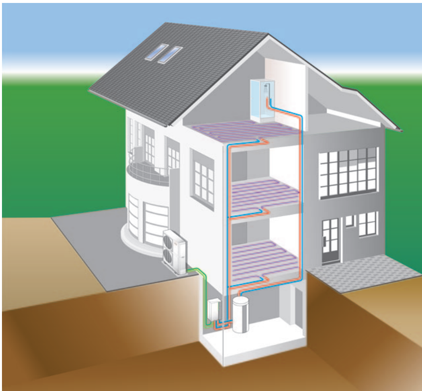
Pompe à chaleur air/eau split
