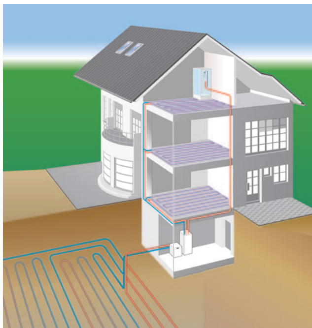
Capteurs géothermiques horizontaux
