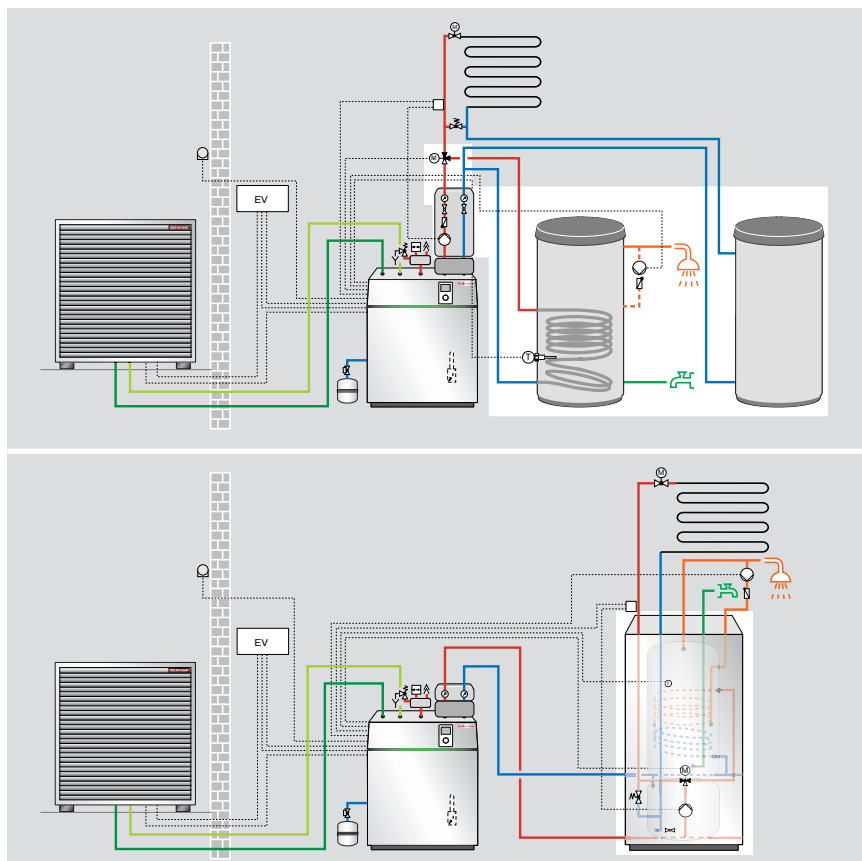
Comparaison d'une installation de pompe à chaleur sans et avec un préparateur multifonction Weishaupt WKS / C
